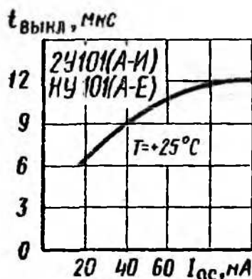
Зависимость времени выключения от тока
